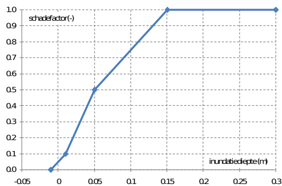
Figuur 4-8 Relatie schadefactor en inundatiediepte voor bebouwing
