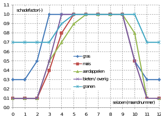
Figuur 4-16 Relatie schadefactor en seizoen voor gewassen
