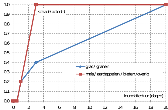
Figuur 4-15 Relatie schadefactor en inundatieduur voor gewassen
